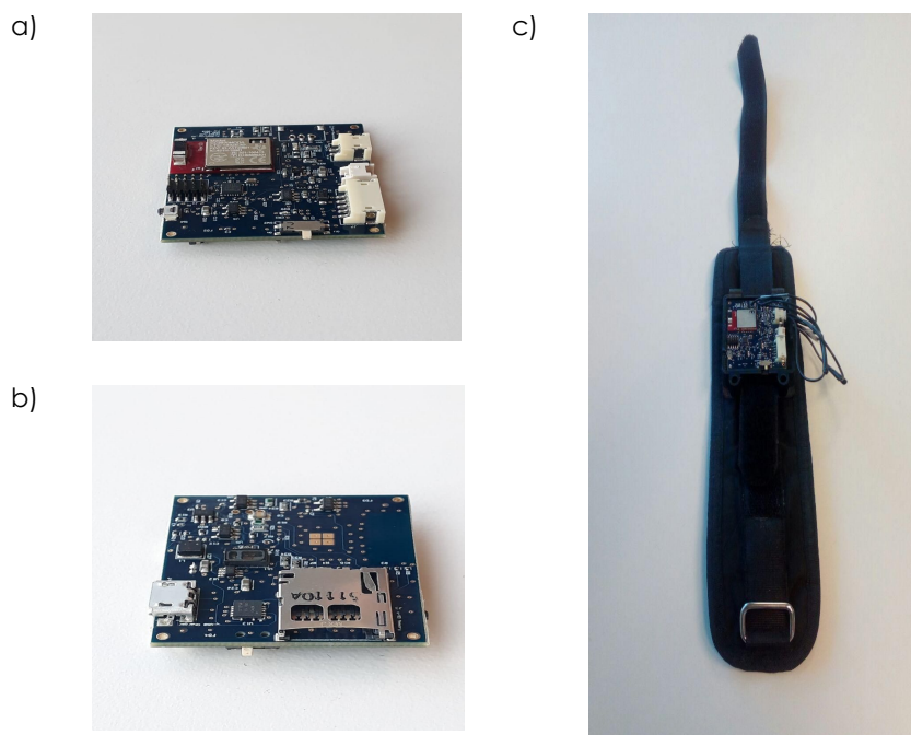
Figura 3: Plataforma de sensado Biomonitor V2.
